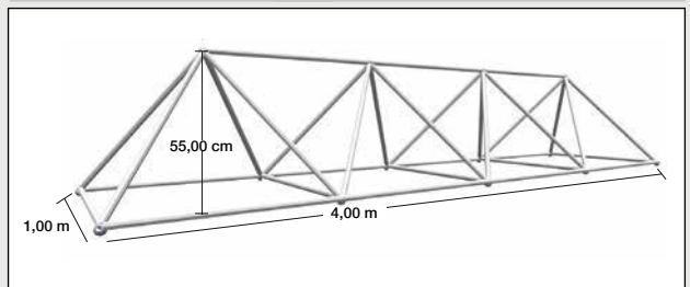
Χωροδικτύωμα
